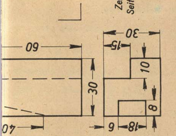
Zeichne die Seitenansicht
