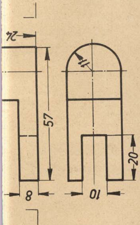
Zeichne Seitenansicht und Ansicht in Richtung A
